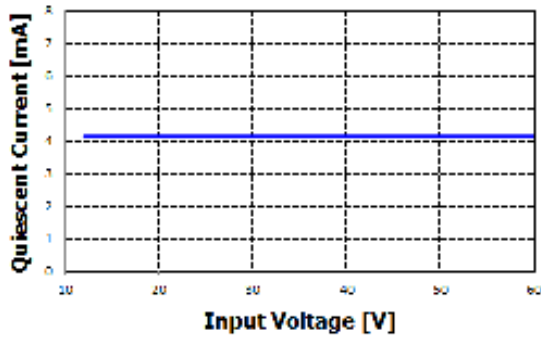
IQ vs. VIN
