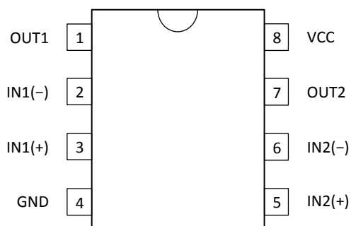
DIP-8
