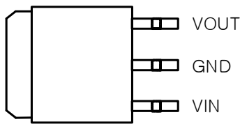
TO263-3L
