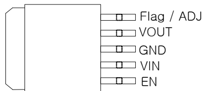
TO263-5L
