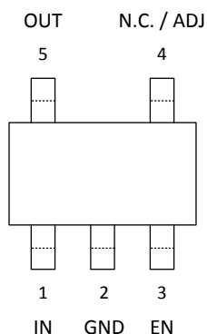
SOT-23-5L
